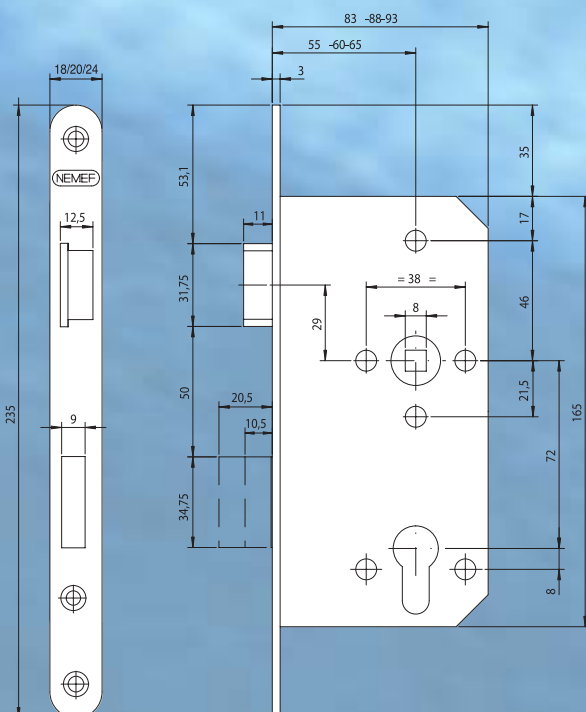
Heavy-duty mortice lock DIN 18251 – part 1, Class III
